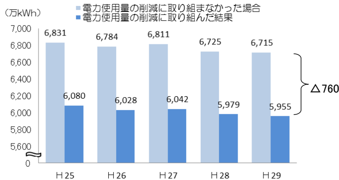
《電力使用量の推移》
